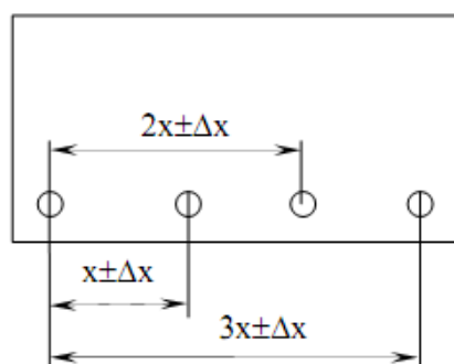
Рис 8.2 Рекомендуемая простановка размеров
